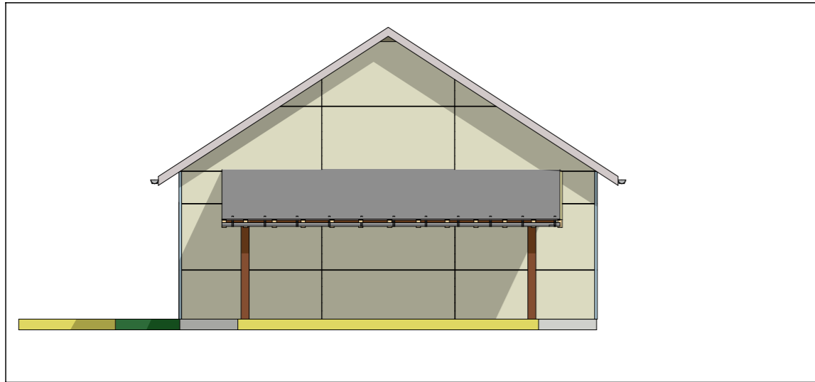
EST1 Façade Est 1:100
