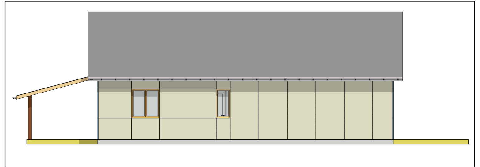
NORD1 Façade Nord 1:100
