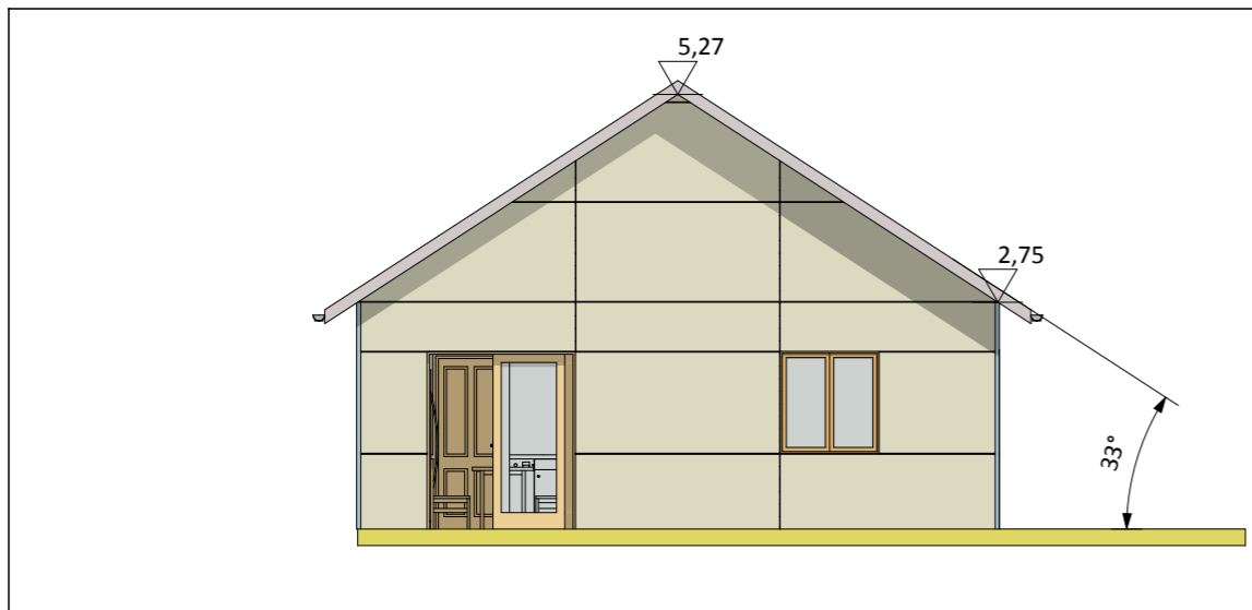
OUEST1 Façade Ouest 1:100
