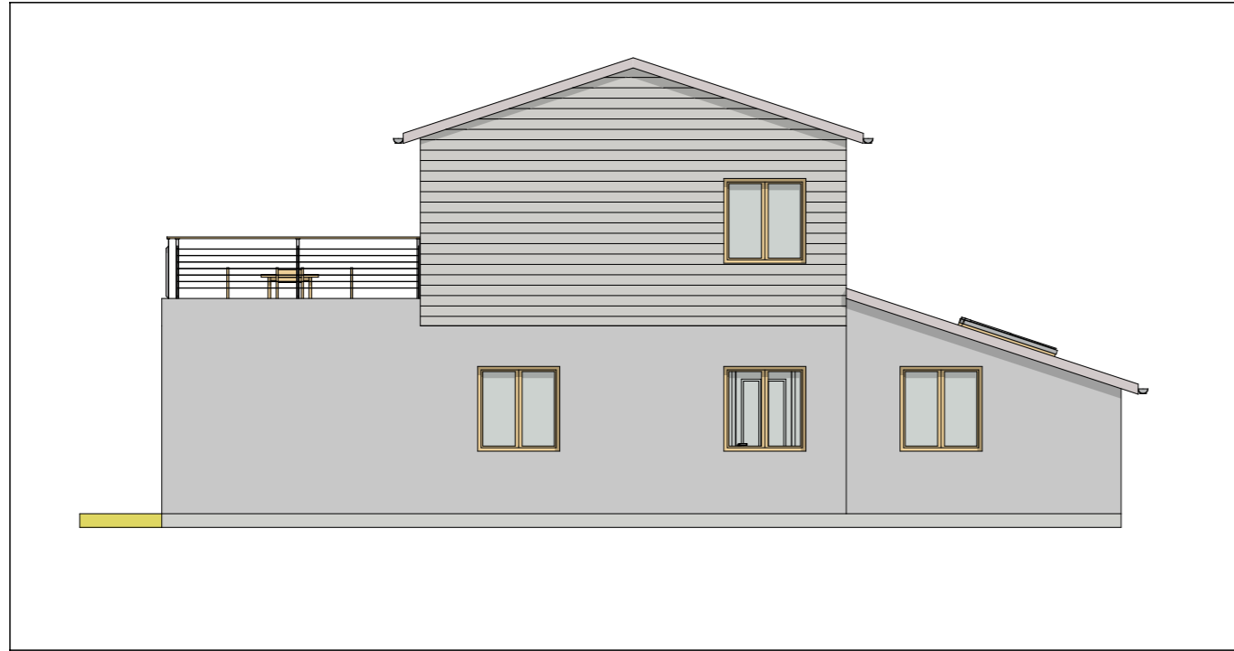
EST Façade Est 1:100
