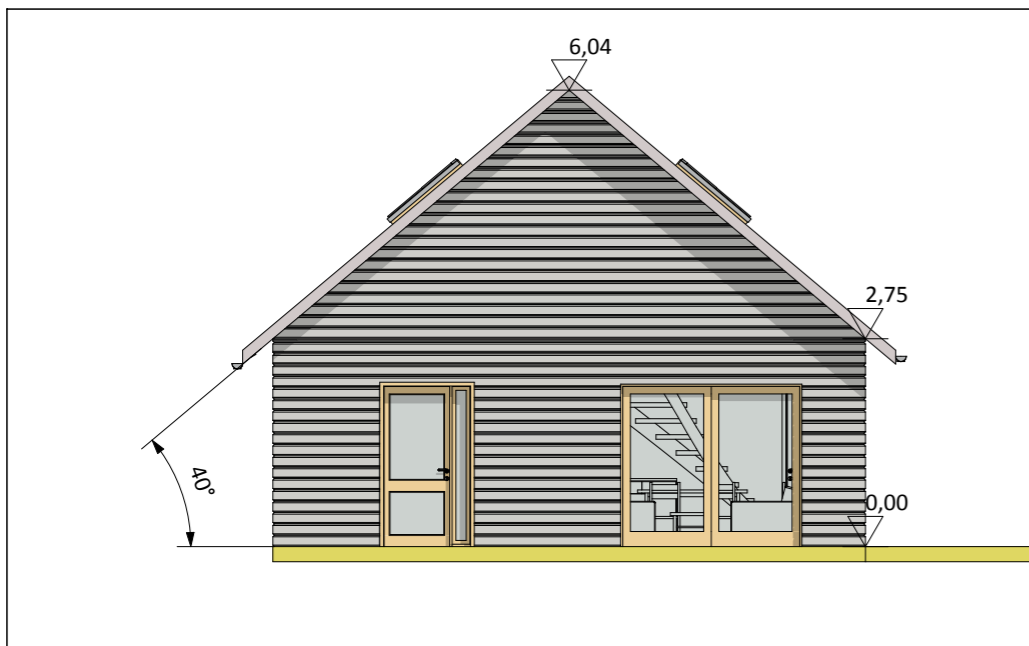
OUEST Façade Ouest 1:100
